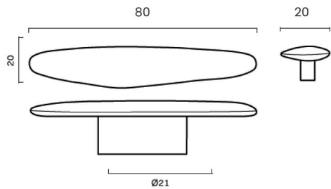
NOBLE T-bar
