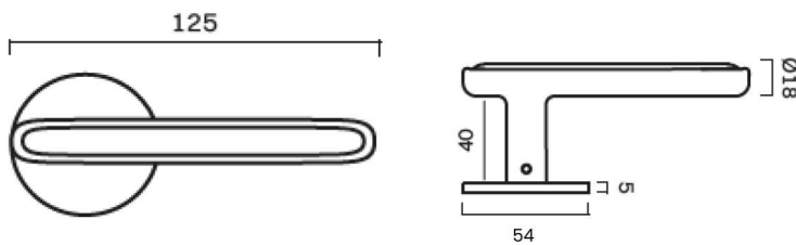
BUTTON door handle
