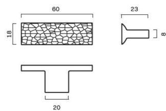
CARVE door handle
