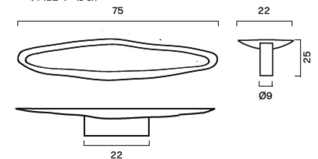
VALE T-bar
