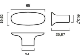
LEAF T-bar
