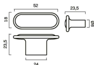
BUTTON T-bar
