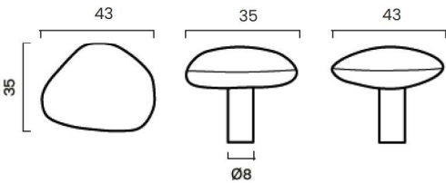
NOBLE knob
