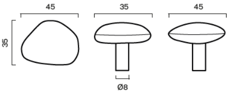
NOBLE knob
