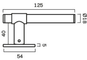
END door handle
