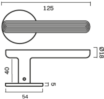
TERRACE door handle
