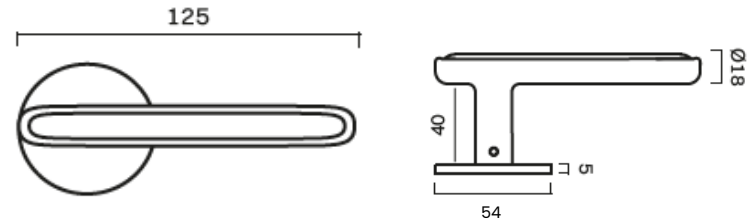
BUTTON door handle
