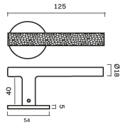
CARVE door handle
