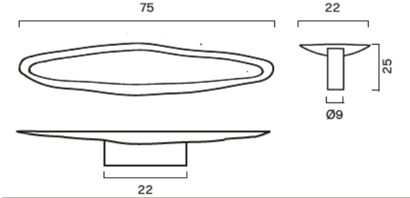
VALE T-bar
